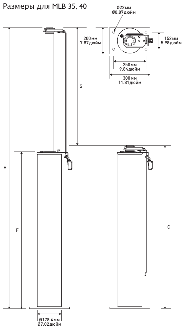
Размеры для MLB 35, 40
