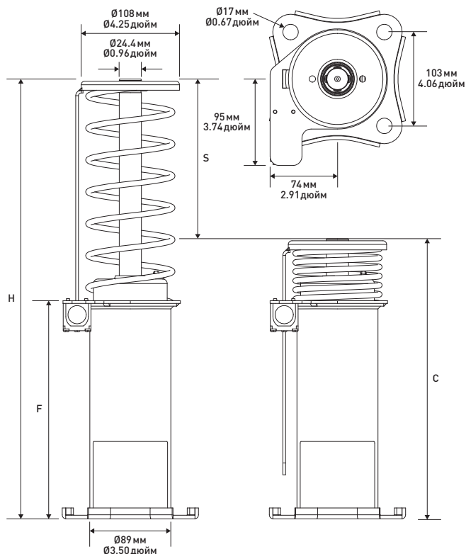
Размеры для LSB 16,18
