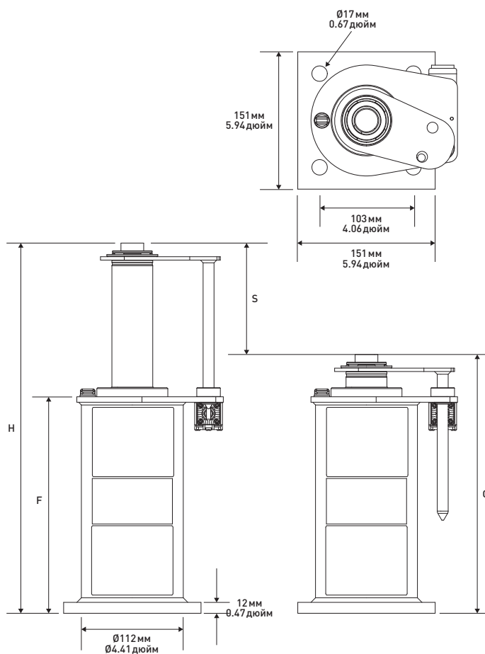
Размеры для MLB 13, 16, 18, 20, 25, 32
