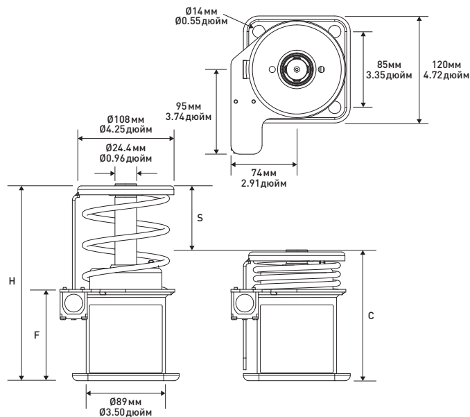
Размеры для LSB 10
